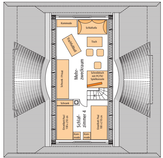
Grundriss Dachgeschoss
